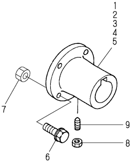
Fig.33 カップリング CUPRING
