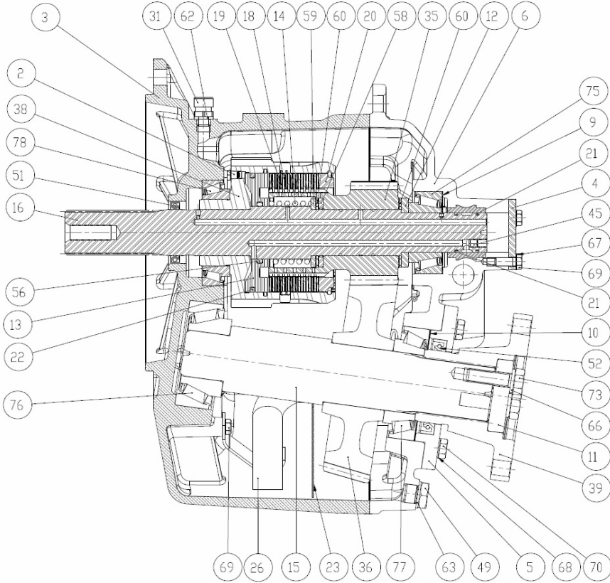
SEZIONE A-A'
